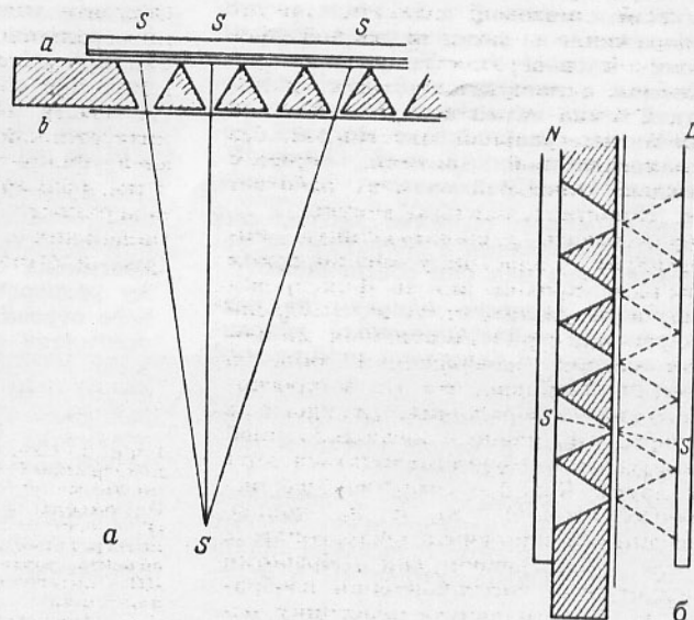
Рис. 3. Схема проверки принципа интегральной фотографии профессором П. П. Соколовым: а — схема съемки; б — схема перепечатки для получения позитива и наблюдения точки S
