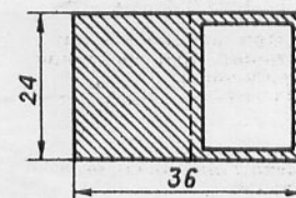
Рис. 2 а. Поле зрения фотографической системы, показанной на рис. 2. Неиспользуемая часть кадра заштрихована
