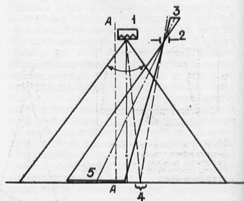
Рис. 2. Условия, при которых исключено возникновение бликов: 1 — вспышка; 2 — объектив; 3 — изображение; 4 — зона блика; 5 — оригинал; АА — плоскость, перпендикулярная оригиналу. Плоскость оригинала параллельна плоскости пленки
