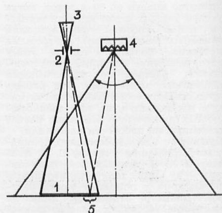
Рис. 1. Возникновение бликов на изображении: 1 — оригинал; 2 — объектив; 3 — изображение; 4 — вспышка; 5 — зона блика. Оптическая ось фотографической системы перпендикулярна плоскости оригинала и проходит через его середину
